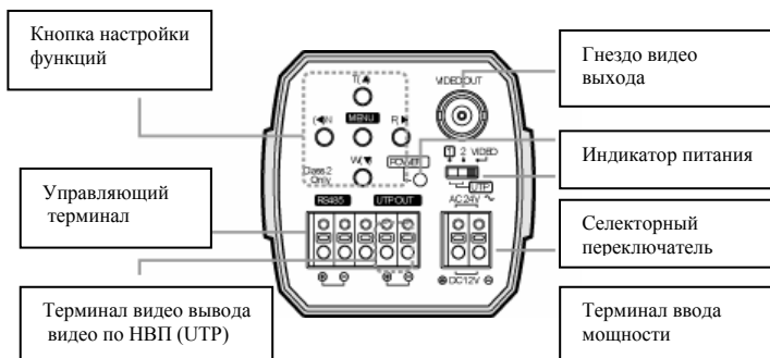
Модель "D" передачи по витой паре (UTP)
