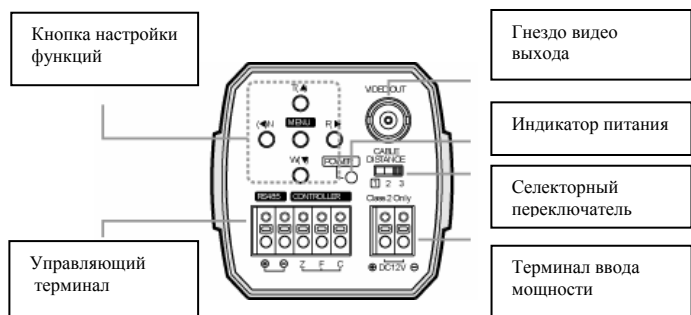
Модель "С" с входом 12В постоянного тока
